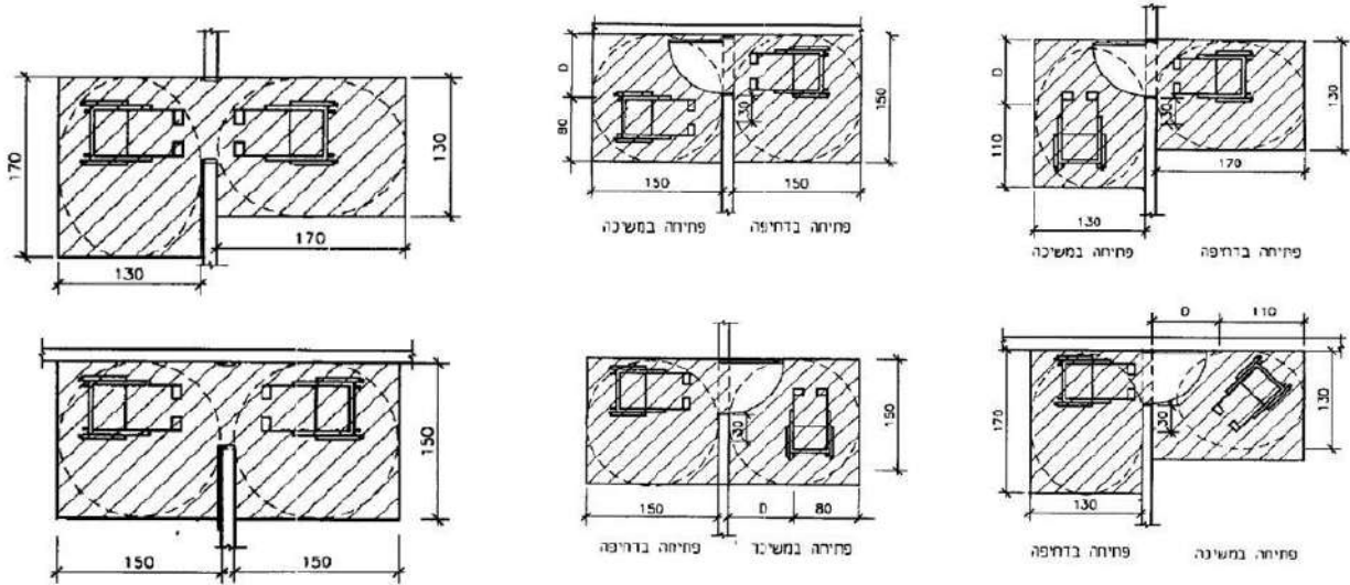
ת"י 1918 חלק 3.1 - משטחי תפקוד לפני דלת סובבת (כל המידות בס"מ)
