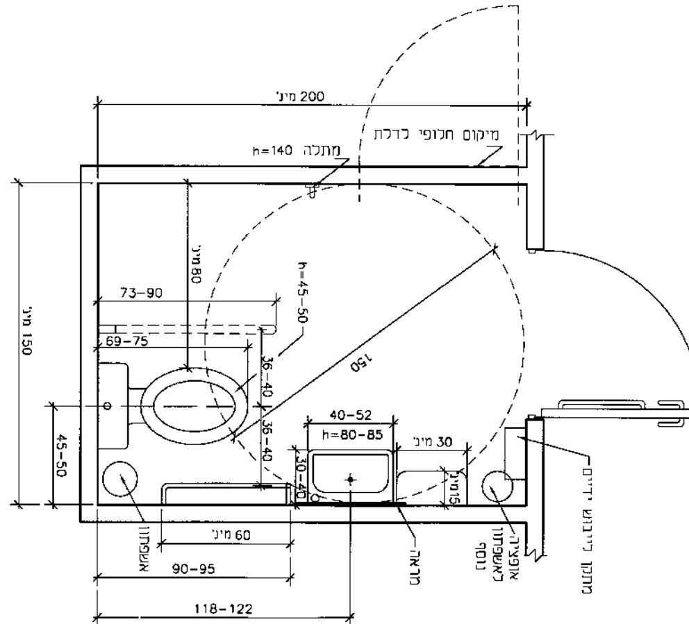
שרטוט המתאר את גודל ומיקום המרכיבים בבית שימוש נגיש, מתוך תקן ישראלי 1918 חלק 3.1
